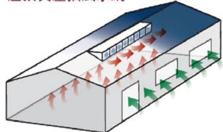
屋頂負壓抽風系統
